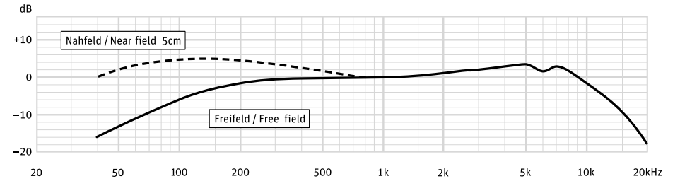
gemessen im freien Schallfeld nach IEC 60268-4 an 10 kOhm Nennlastimpedanz measured in free-field conditions (IEC 60268-4) into 10 kohm rated load impedance
